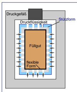
Isostatisches Pressen
