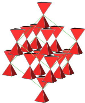
Cristobalit (> 1470 °C)
