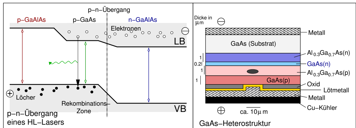
HL-Laser: E-Niveaus und schematischer Aufbau
