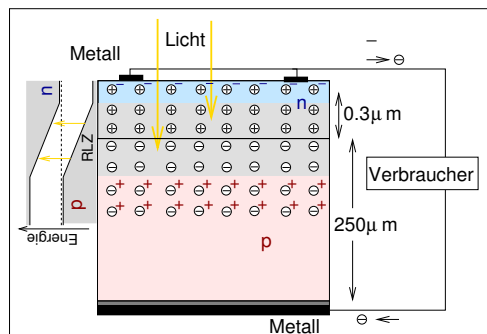
Photovoltaik: Solarzelle
