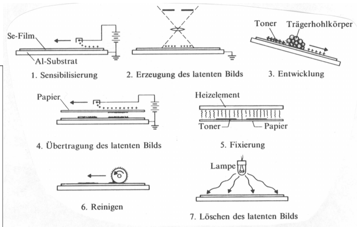
Xerographie
