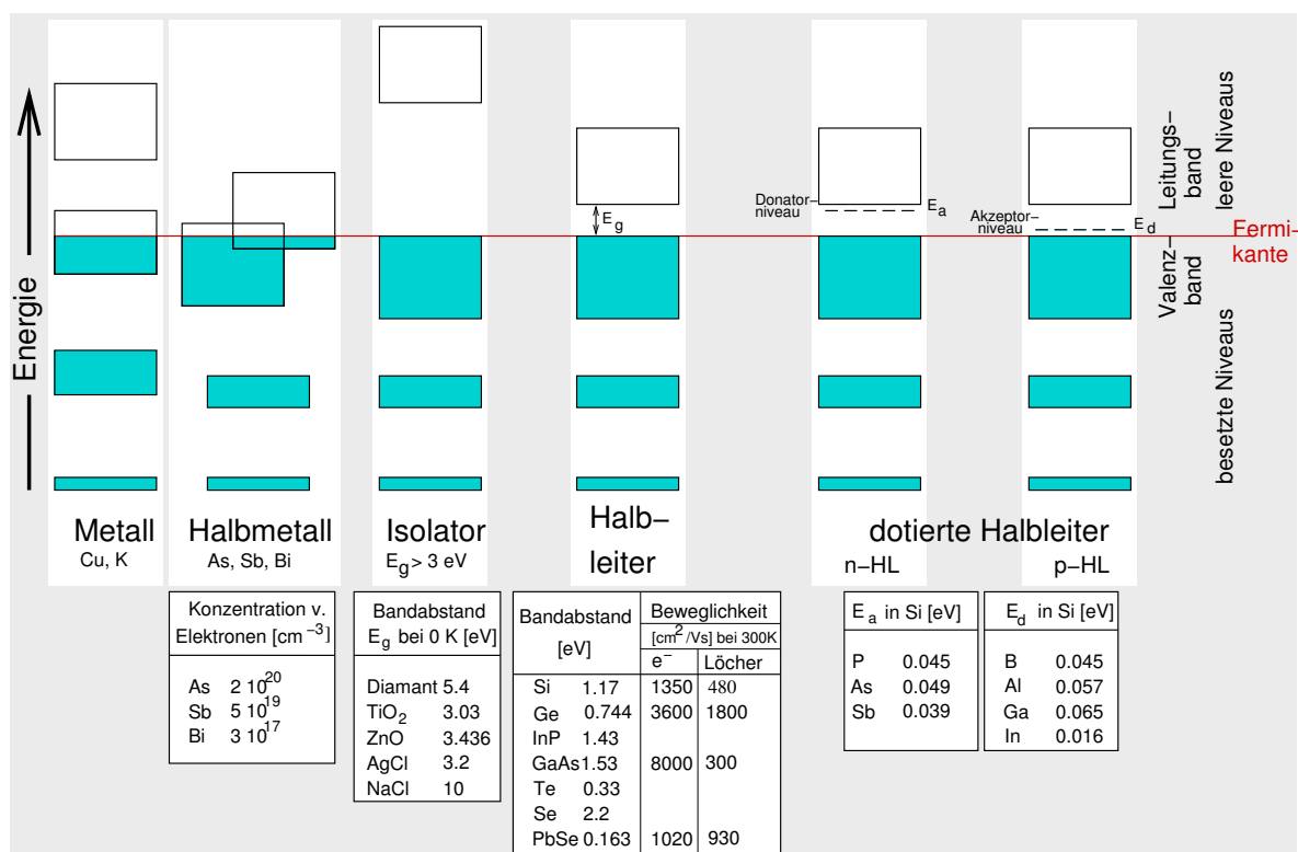
vereinfachte Zustandsdichten verschiedener Festkörper
