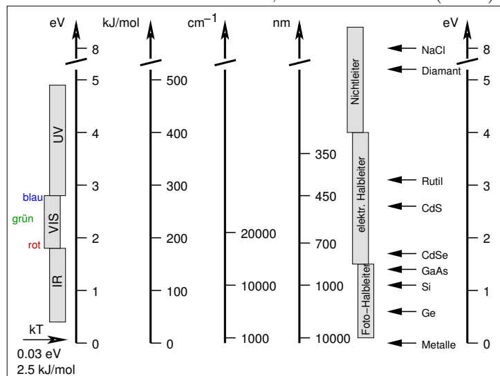
Energieskala und Bandlücken
