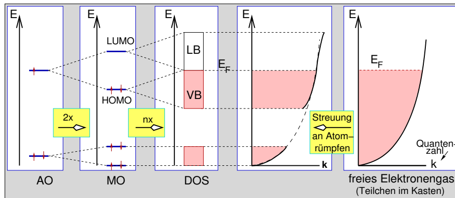
Bandstruktur, Zustandsdichte (DOS)
