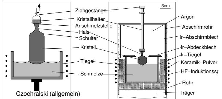
Czochralski-Verfahren (allgemein und für Granate)
