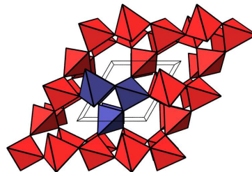
Struktur von \alpha -Quarz
