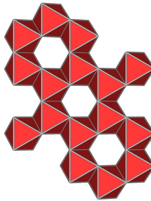
von Korund
