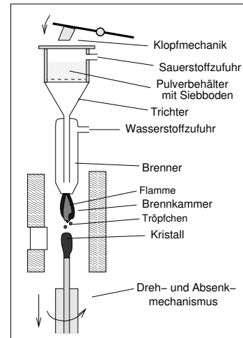
Verneuil-Verfahren
