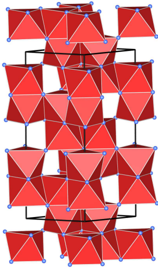
Struktur
