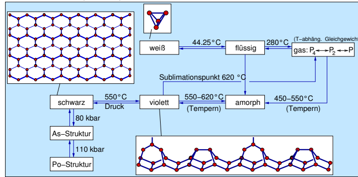
Polymorphie von Phosphor
