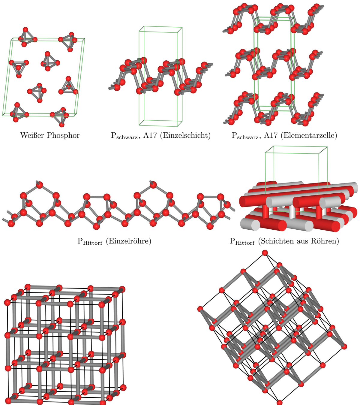
Zusammenhang zwischen α-Po und As grau (A7) (zwei verschiedene Ansichten)
