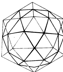
h) Ikosidodekaeder
