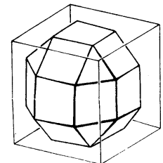
f) Rhombenkuboktaeder
