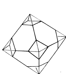
b) abgest. Oktaeder
