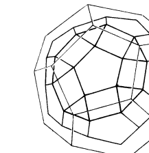
m) Rhombenikosidodekaeder
