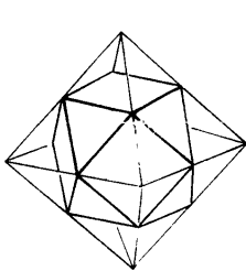
g) Kuboktaeder
