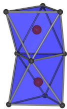
Rb_9O_2 Cluster als Bauelemente der Suboxide
