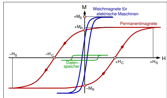
Hysteresekurven (nach Anwendungsbereich)
