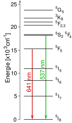
Termschema von \text{Ho}^{3+}
