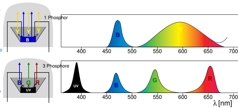
Aufbau weisser LEDs
