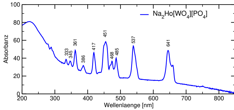
UV/VIS-Spektrum von \text{Na}_2\text{Ho}[\text{WO}_4][\text{PO}_4]
