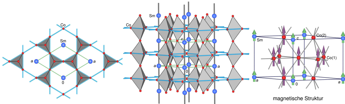
Kristallstruktur von \text{SmCo}_5 ( \text{CaCu}_5 -Typ)
