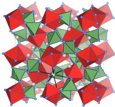
Granat-Struktur
