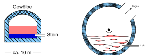
Konverter (schematisch)
