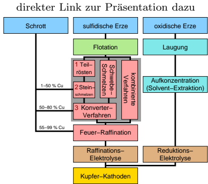
Übersicht Cu-Gewinnung
