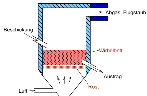
Wirbelschichtreaktor (schematisch)
