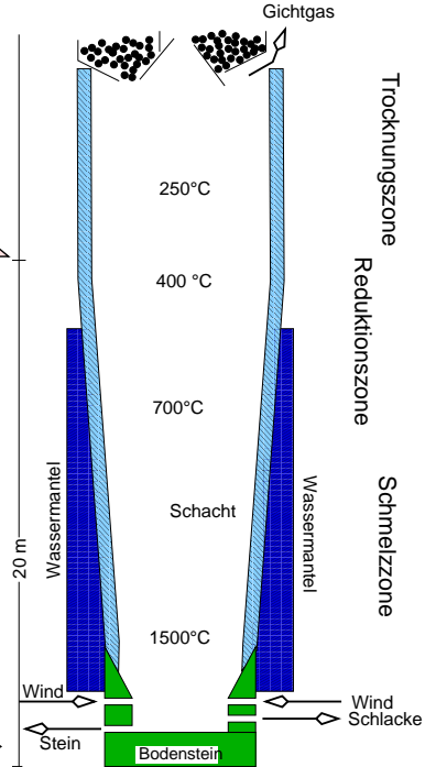
Wassermantelofen
