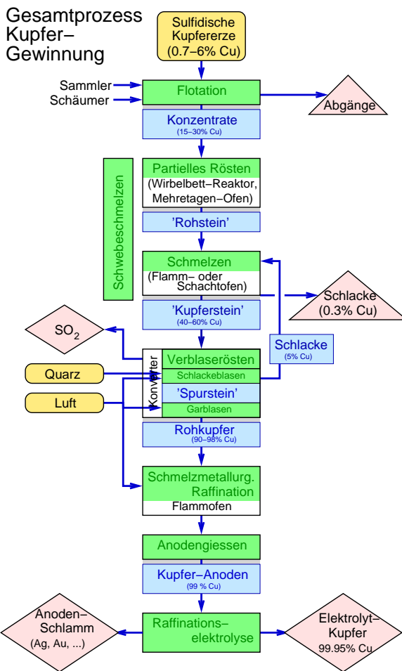
Übersicht Cu-Gewinnung
