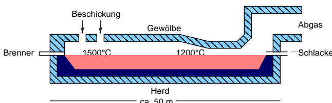
Flammofen (schematisch)
