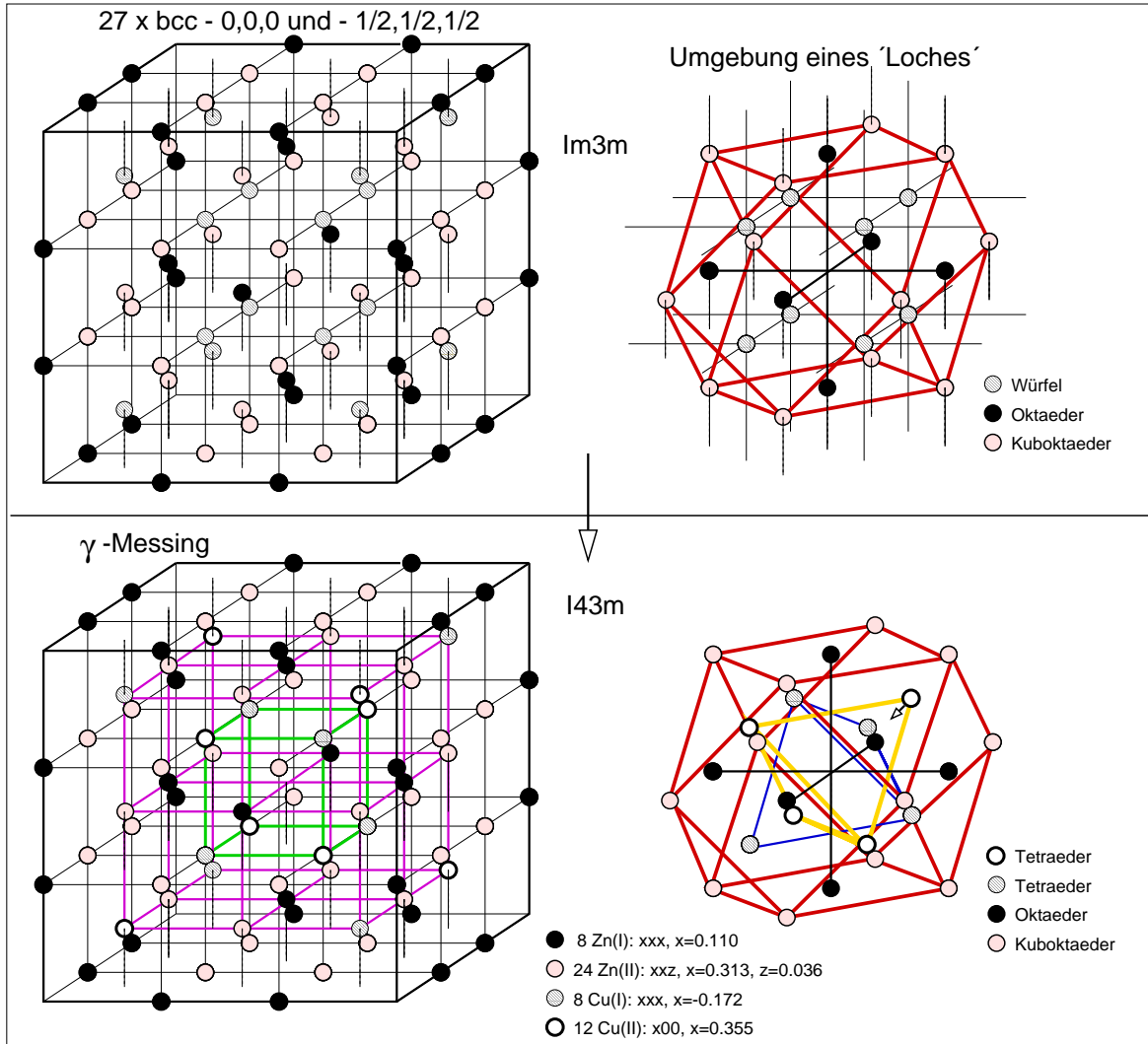
Struktur von \gamma -Messing
