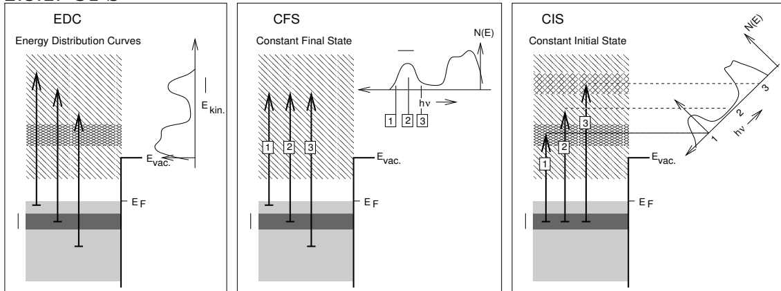
Meßtechniken bei der UPS-Spektroskopie
