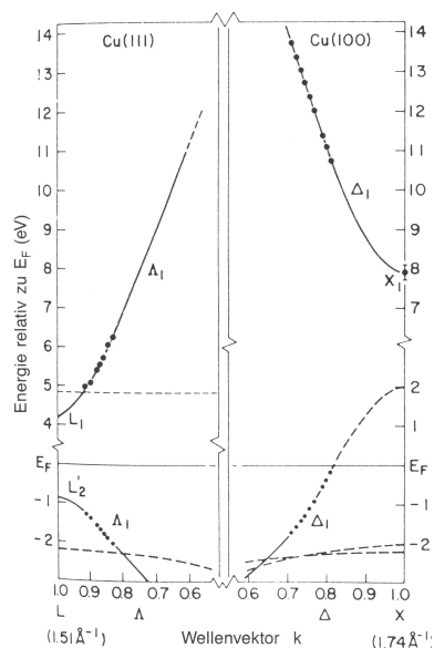
Bandstruktur von Cu mit Meßpunkten aus CIS-Spektren (s.o.)
