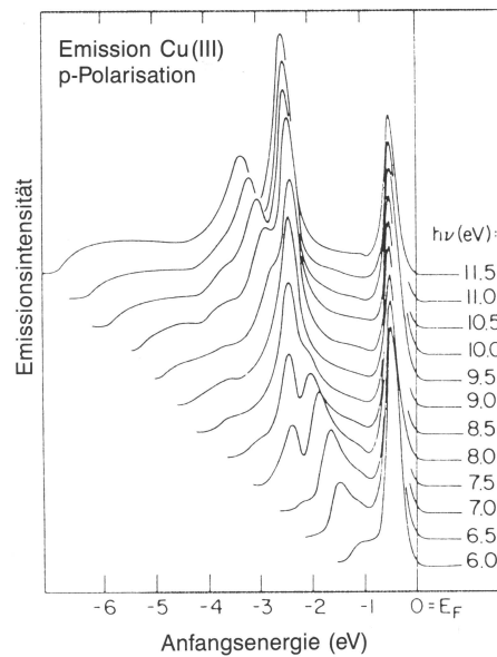
CIS-Messungen der Cu(111)-Oberfläche
