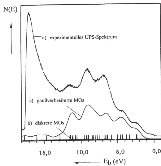
UPS-Spektrum von Diaminobenzol auf einer Si(100)-Oberfläche
