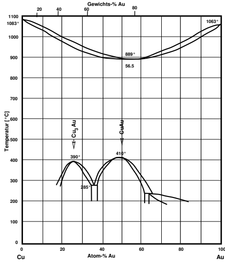
Phasendiagramm Cu-Au
