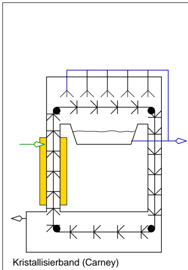
Bauarten von Kristallisationsapparaten für die Lösungs- und Schmelzkristallisation
