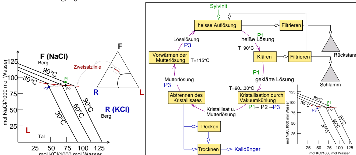
Aufbereitung sylvinitischer Rohsalze
